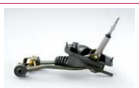
96 Radiace ústrojenstvo STI (5MT) C1010AG001 W Pre kratšie dráhy radenia, rýchlejšie a precíznejšie radenie. *Nie pre vozidlá s redukčnou prevodovkou Dual-Range.
